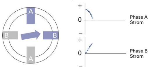
Abb. 14 Mikroschrittbetrieb bei einem 2-Phasen-Schrittmotor mit quasi sinusförmigen Stromverläufen.
